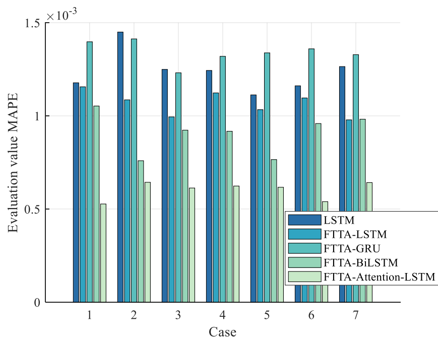
(b) MAPE
