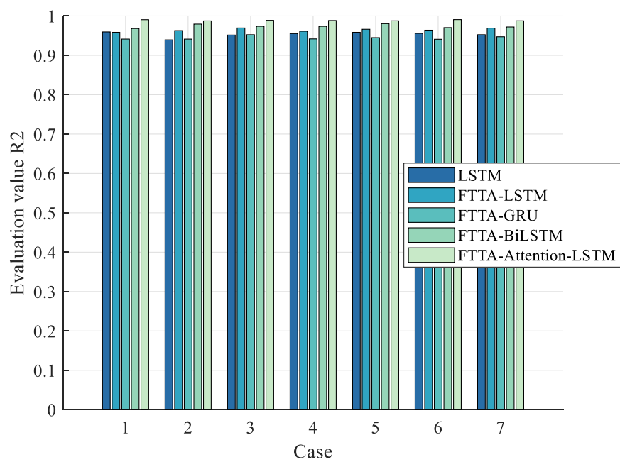
(d) R^2
